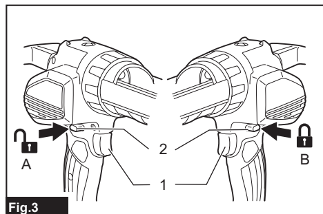
Fig.3 ► 1. Gâchette 2. Bouton de verrouillage de la gâchette
